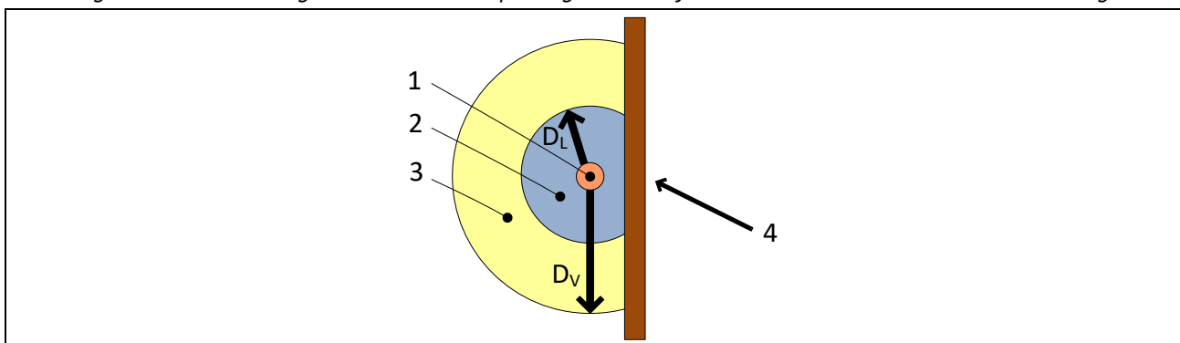
Figuur 2.29. Voorstelling van de zone onder spanning en de nabijheidszone met isolerende bescherming
