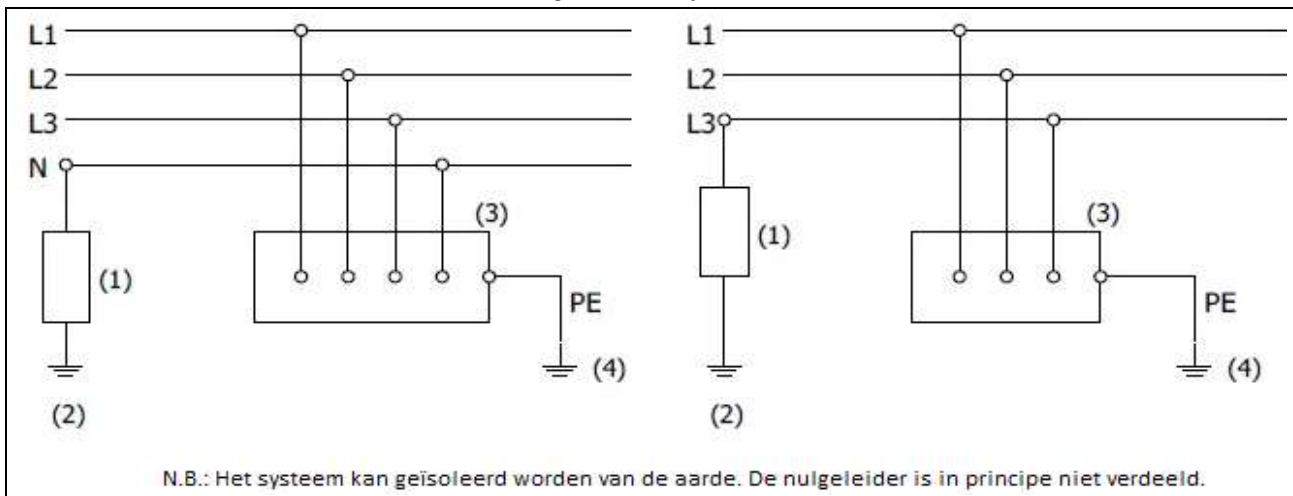
Figuur 2.5. IT-systeem
