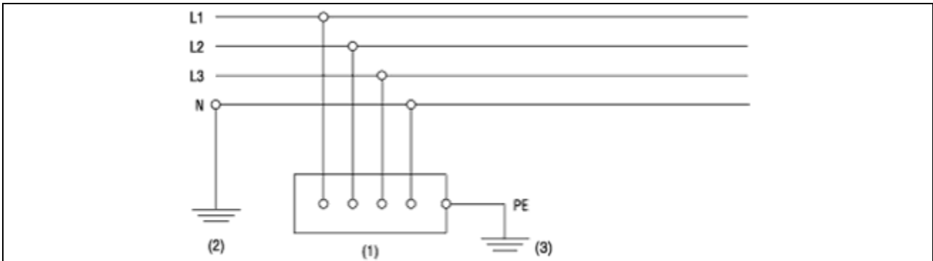
Figuur 2.4. TT-systeem
