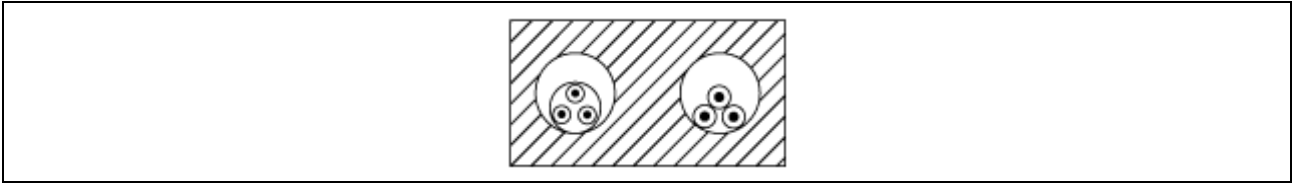
Figuur 2.18. Plaatsingswijze «holle blok»
