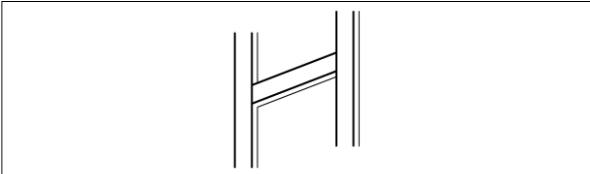
Figuur 5.21. Plaatsingswijzen van elektrische leidingen – Achter wandpanelen
