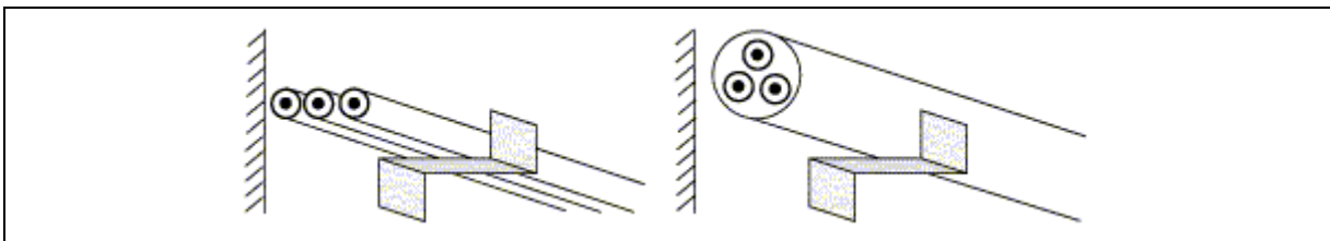
Figuur 5.10. Plaatsingswijzen van elektrische leidingen – Haken
