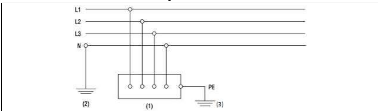
Figuur 3.2. TT-net
