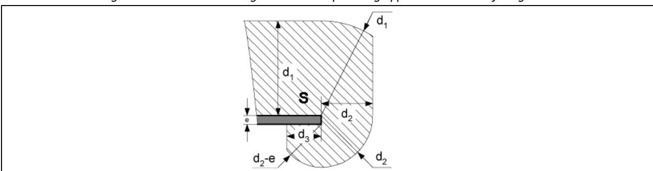
Figuur 2.6. Genaakbaarheidsgebarit: het verplaatsingsoppervlak is natuurlijk begrensd
