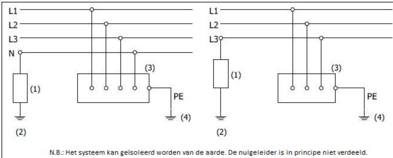
Figuur 3.3. IT-net
