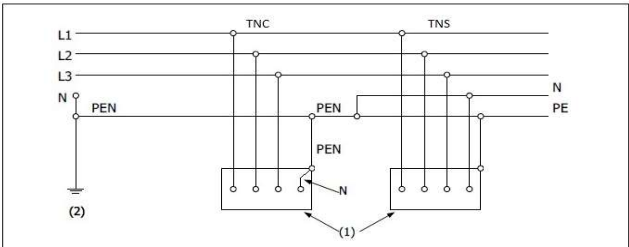
Figuur 2.3. TN-C-S-systeem
