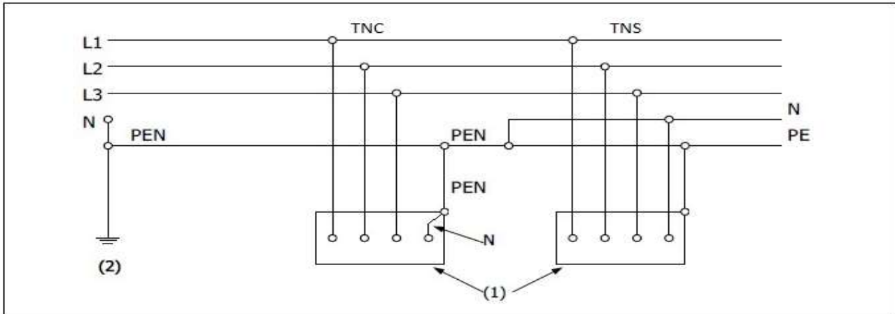
Figuur 3.1. TN-C-S-net
