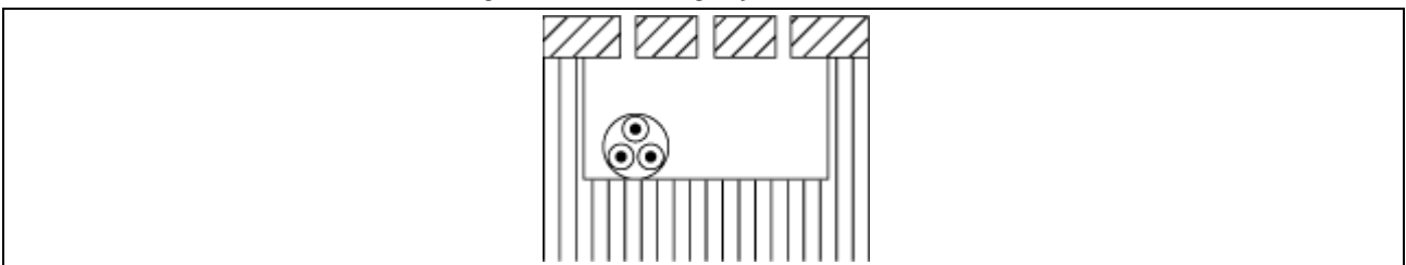
Figuur 2.19. Plaatsingswijze «kabelkanaal»
