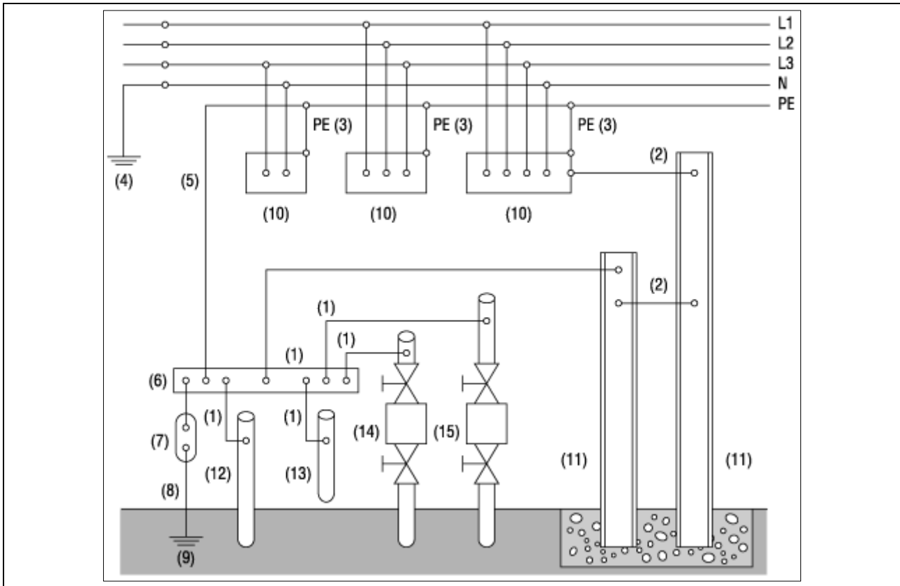
Figuur 2.11. Aardingsinstallatie
