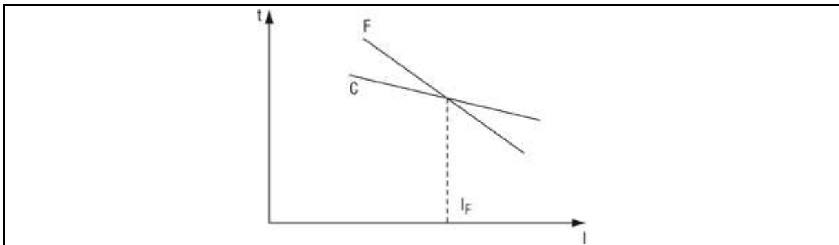
Figuur 5.43. Keuze van de beschermingsinrichting tegen kortsluitingen bij smeltveiligheden
